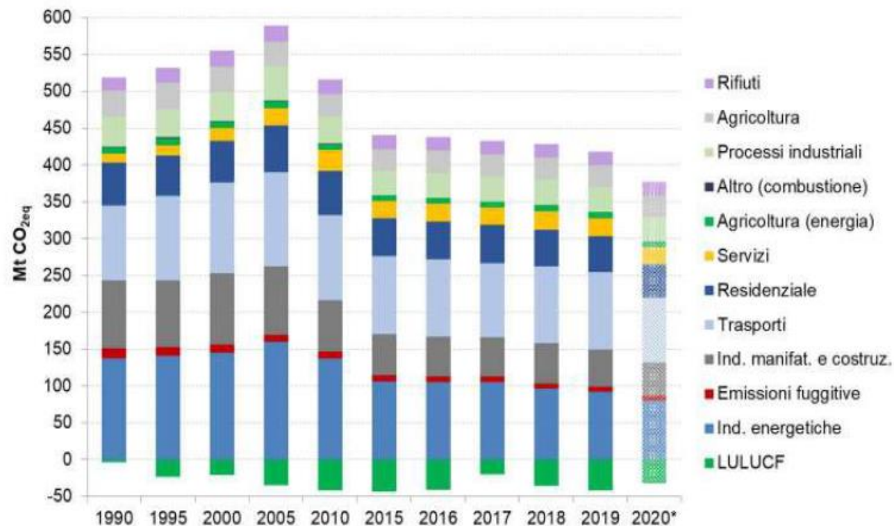
Figura 1.12 – Emissioni di gas ad effetto serra per settore. Il settore agricoltura e pesca è riportato come agricoltura e le emissioni sono distinte da combustione (energia) e da processo. Per il 2020 sono riportate le stime preliminari elaborate da ISPRA.
