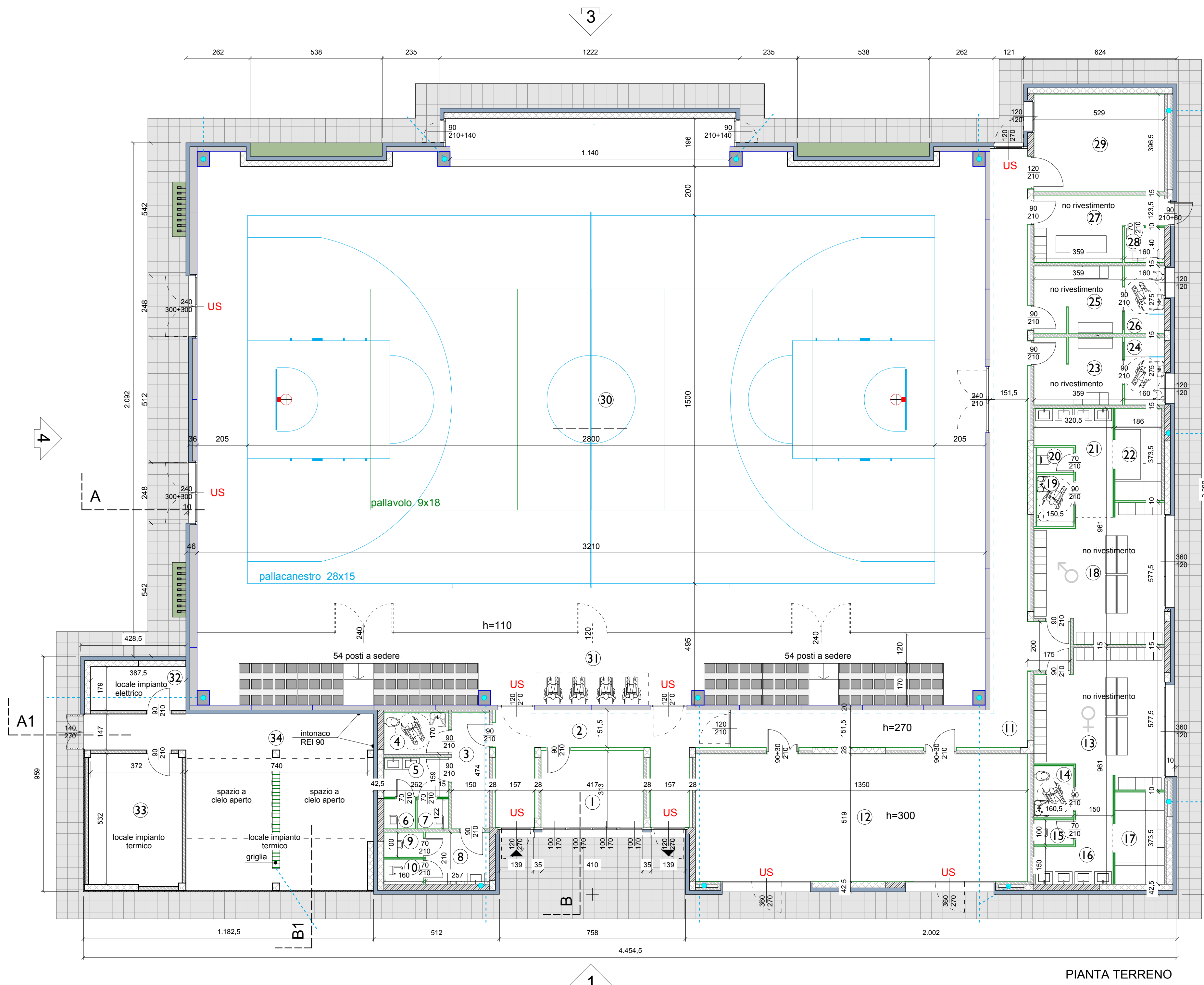
PIANTA TERRENO
