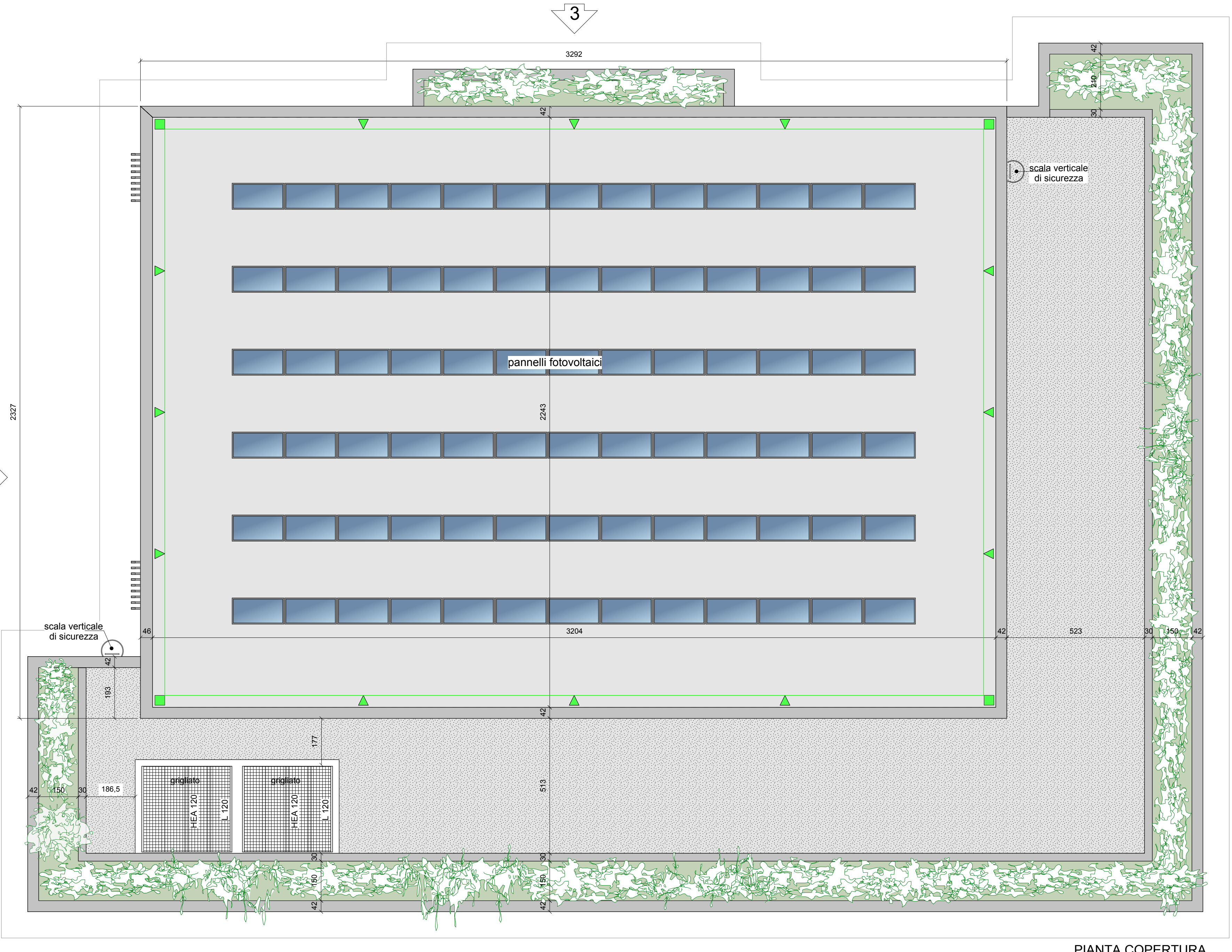
PIANTA COPERTURA
